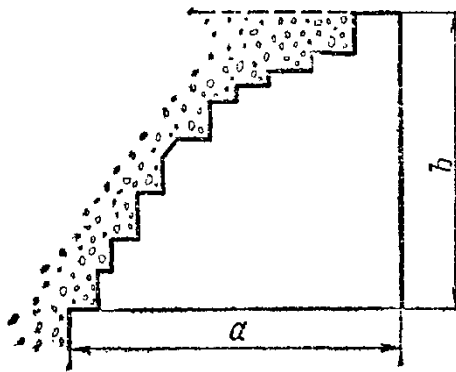
Рис. 4. Наружный карниз а - относ карниза; - высота карниза
