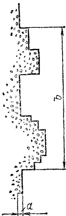
Рис. 5. Стенная тяга а - относ тяги; - высота тяги
